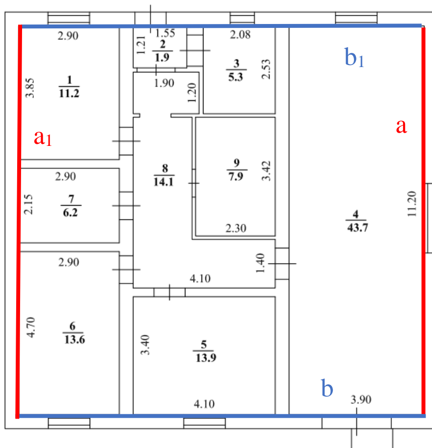
Рис. 14. Линейные измерения для расчета СКП площади здания 6.14.5. Определение СКП площади здания по СКП внешнего контура здания и СКП наружных стен
