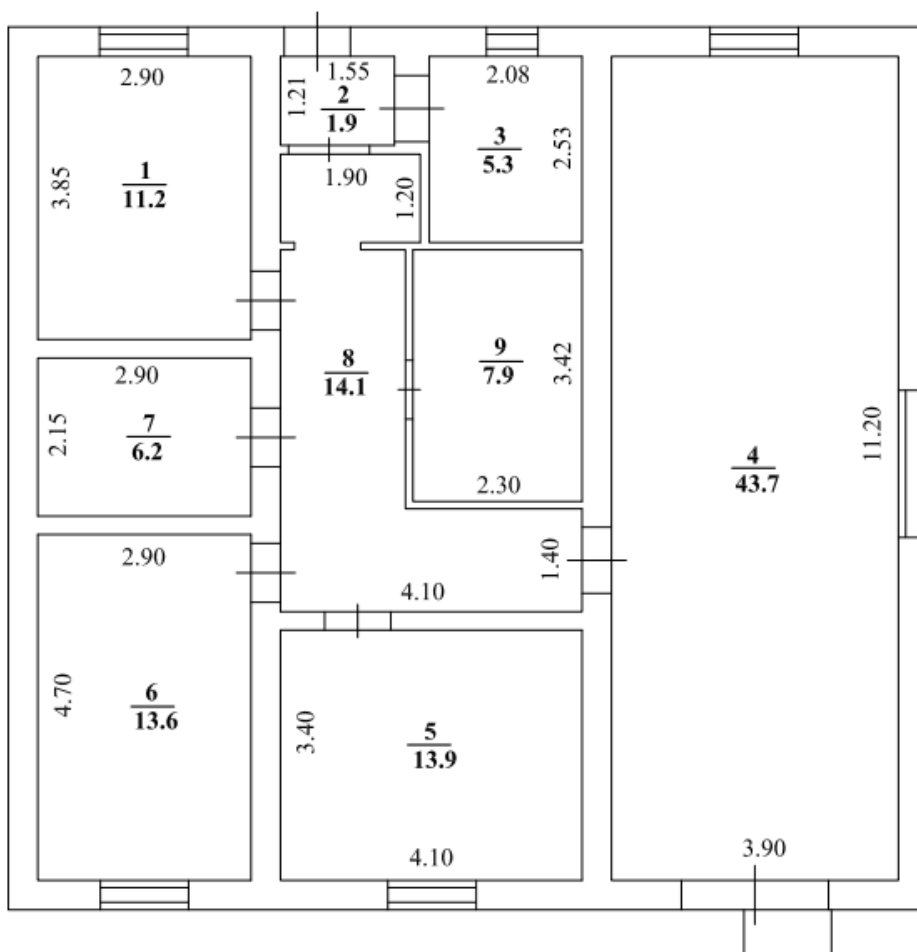
Рис. 10. Поэтажный план здания – объекта кадастровых работ
