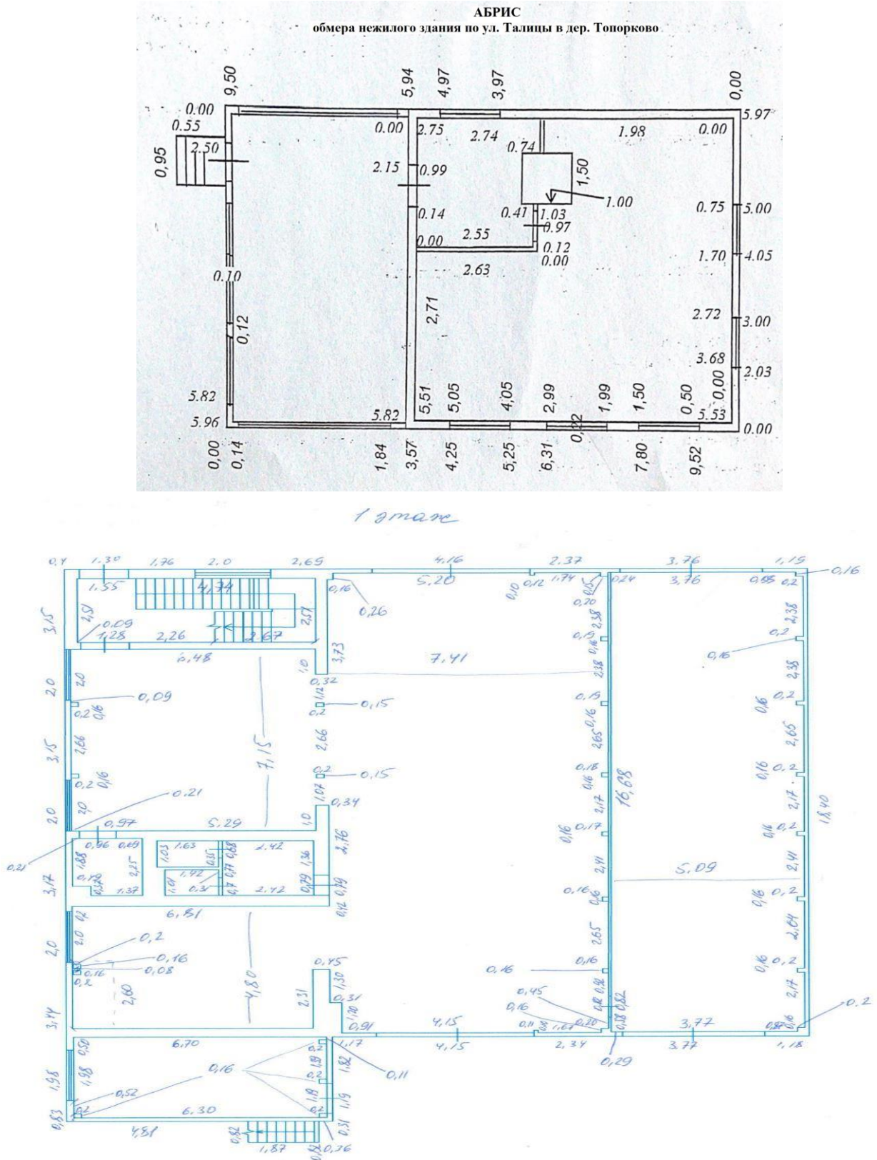
Рис. 20. Примеры абрисов нежилого здания
