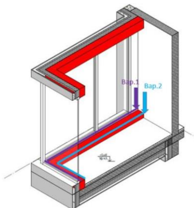
Рис. 8. Особенности подсчета площади здания при наличии напольных систем отопления.
