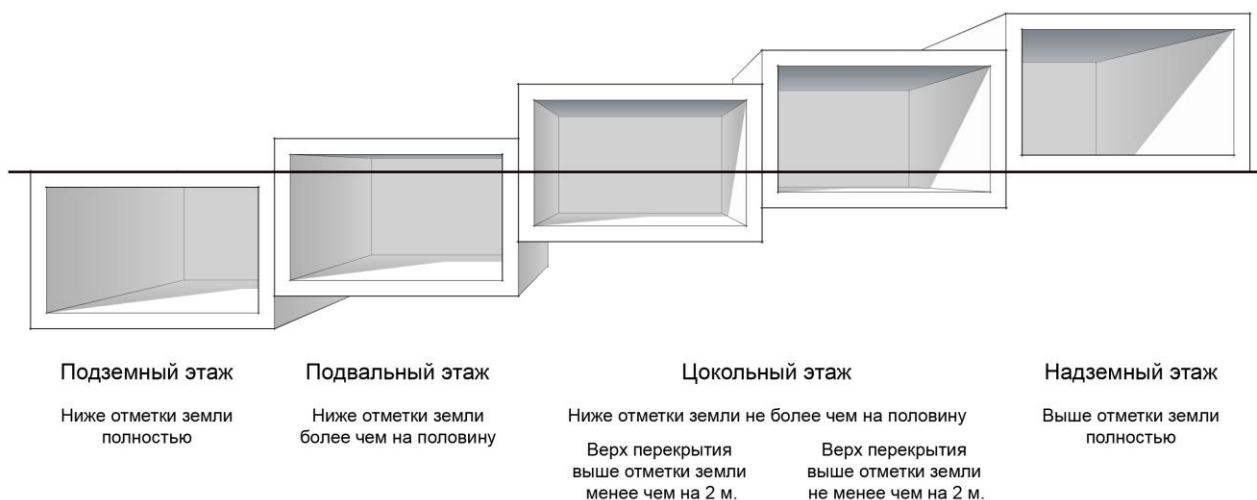
Рис. 5. Сравнение подземного, подвального, цокольного и надземного этажа 2
