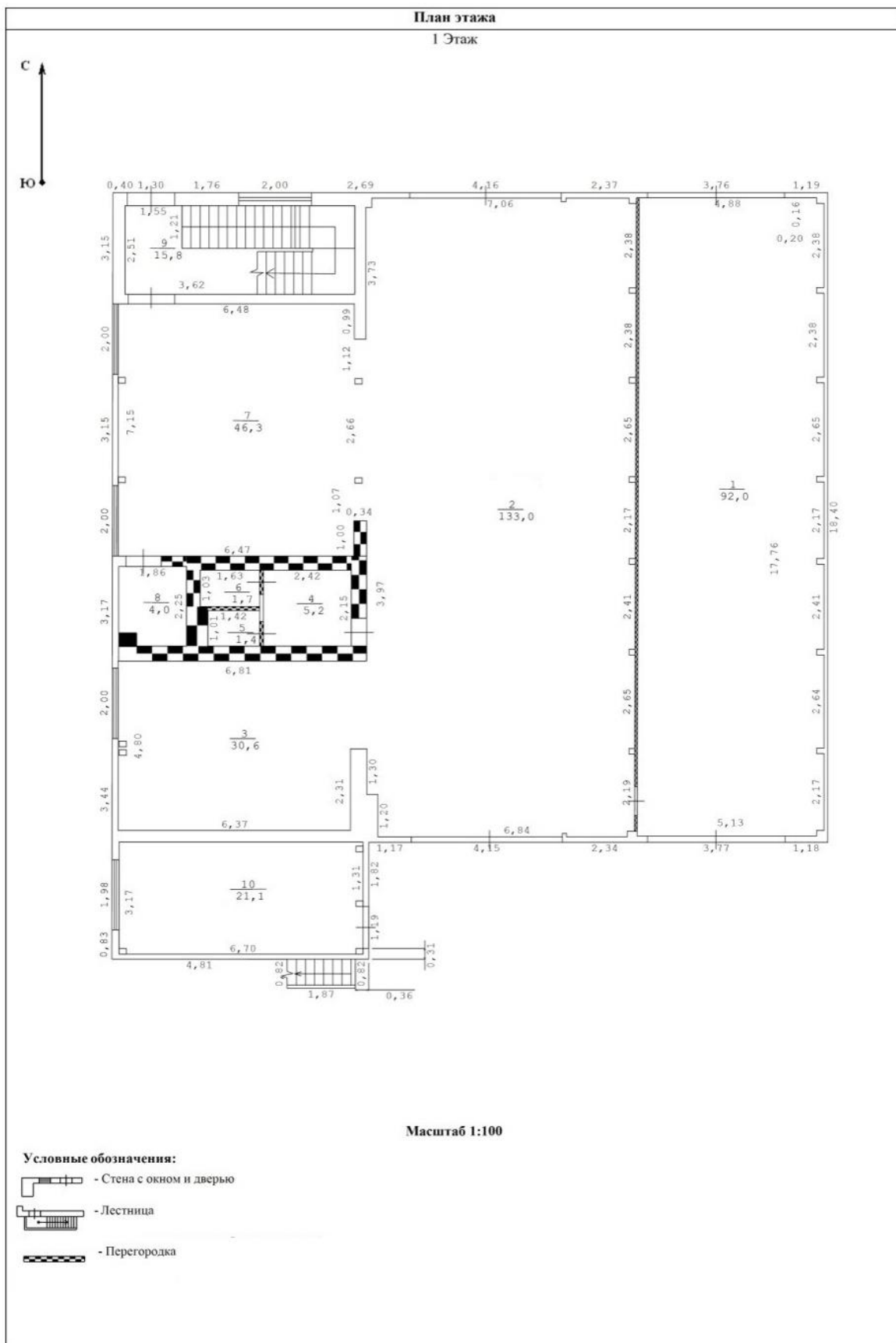
Рис. 21. Пример оформления Плана этажа нежилого здания в техническом плане
