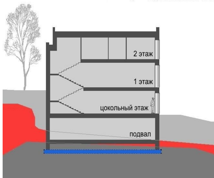
Рис. 6. Пример определения наименования этажей общественного здания на склоне 3
